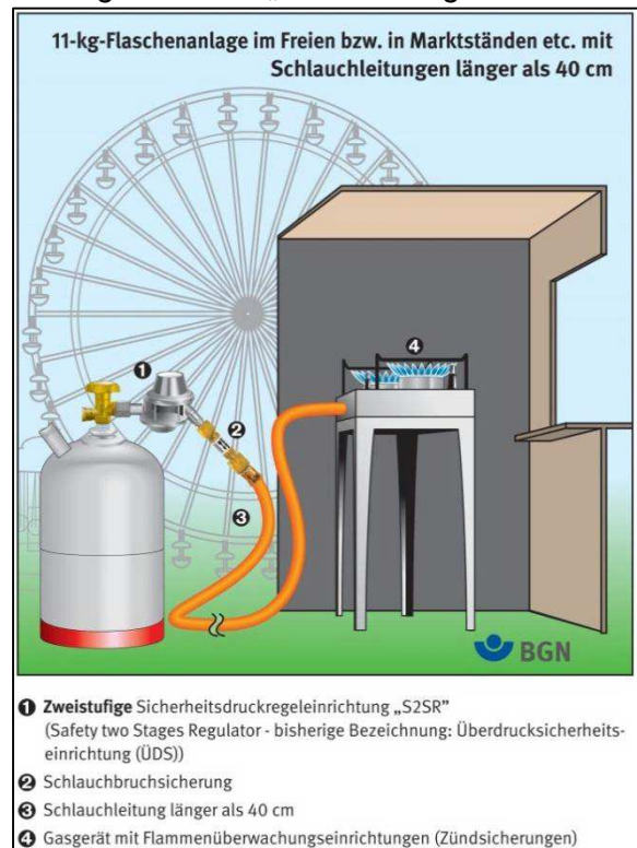
Bild 1 Beispielhafte Flüssiggasanlage
